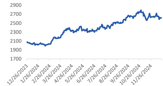
Vàng (USD/oz)
